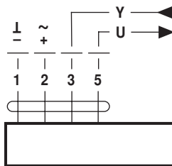
NM24A-SR.. NM24A-MF..
